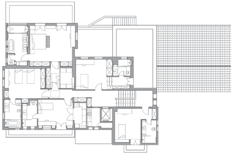
κάτοψη ορόφου
