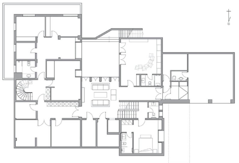
κάτοψη υπογείου
